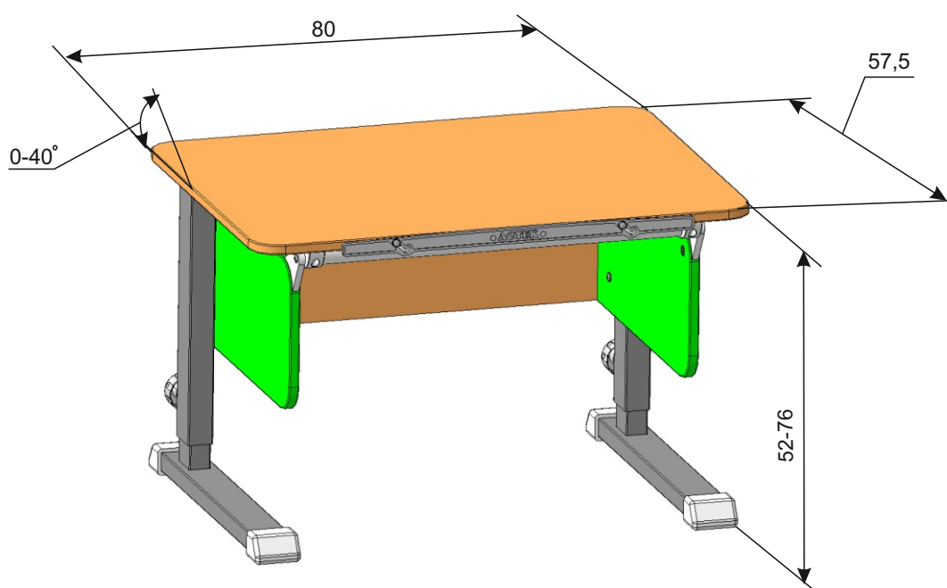
Рисунок 1- Основные размеры
