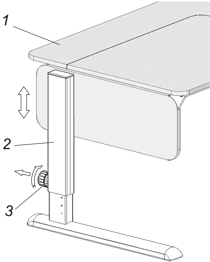
Рисунок 2- Регулировка высоты стола: 1- корпус стола, 2- опора, 3- фиксатор
