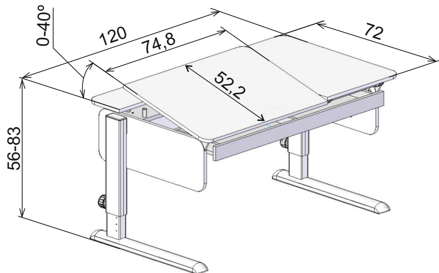
Рисунок 1- Основные размеры стола, см
