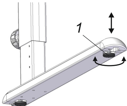
Рисунок 4- Регулировка опор
